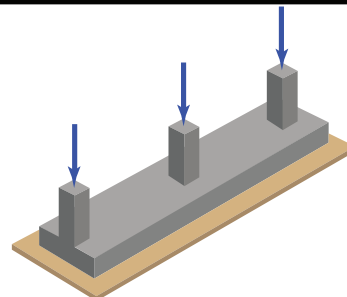
شالوده نواری
