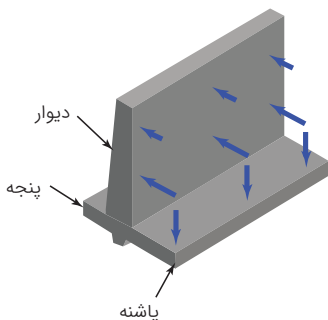
دیوار حائل
